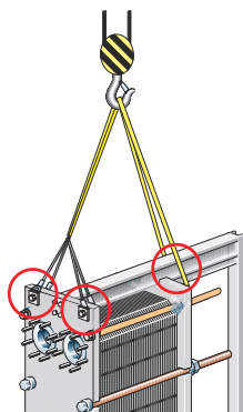
Figur 7: Løfte Semisveiset MK15.
