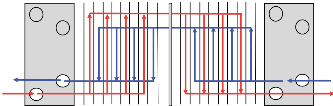
Figur 3: Eksempel på oppsett med flere passeringer.
