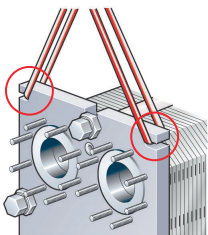
Figur 5: Løfte M6, M10 og T10.
