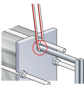
Figur 6: Løfte M6, M10 og T10.
