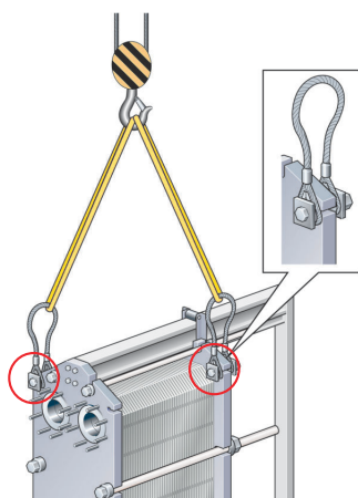
Figur 8: Løfte Semisveiset TK20 og Semisveiset T20.
